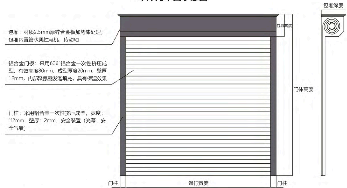
车库门平面示意图
