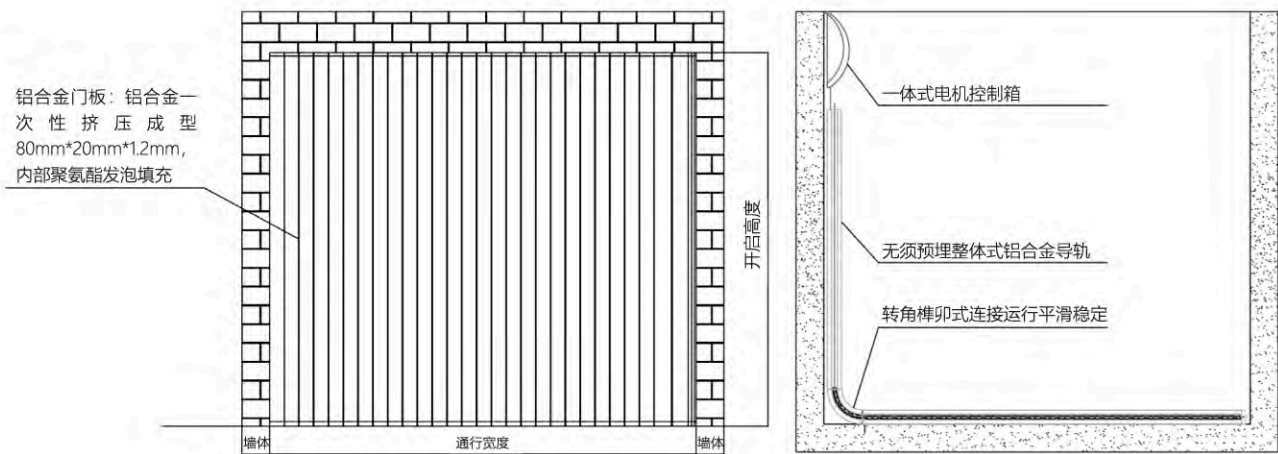
车库门平面示意图
