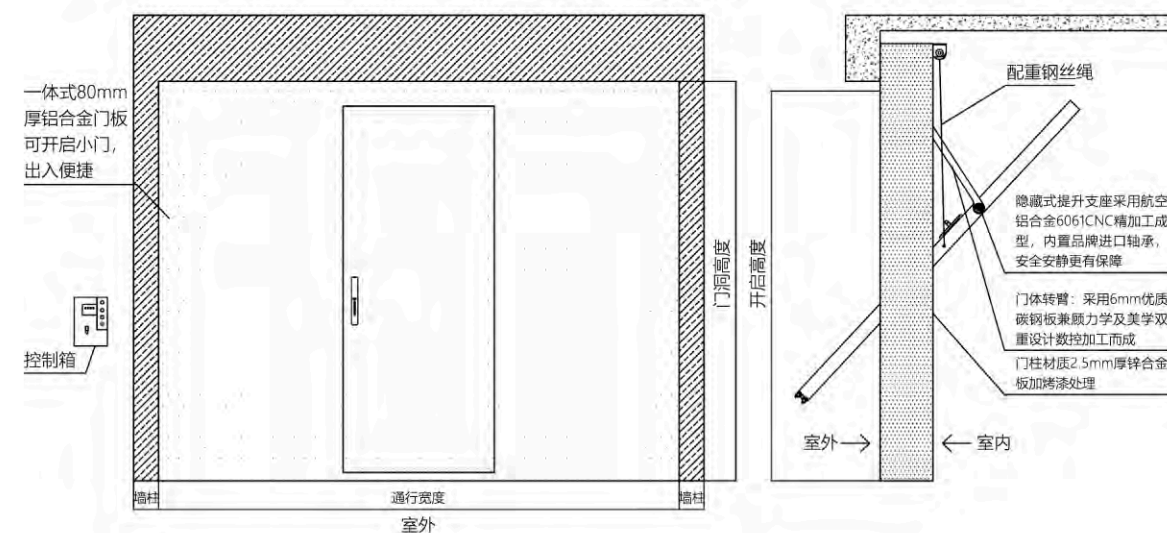
车库门平面示意图
