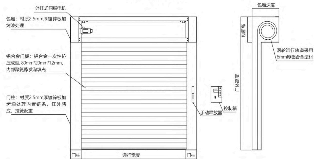
车库门平面示意图
