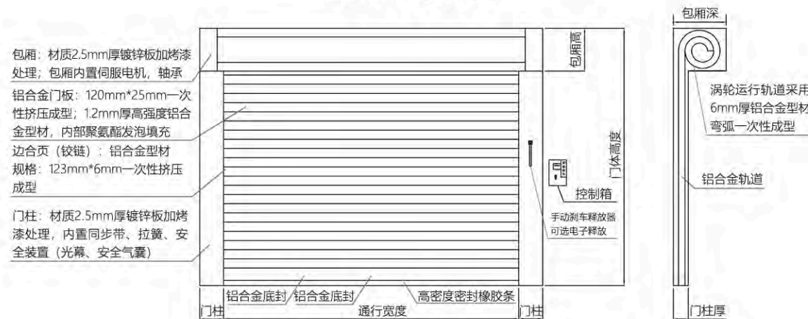
车库门平面示意图
