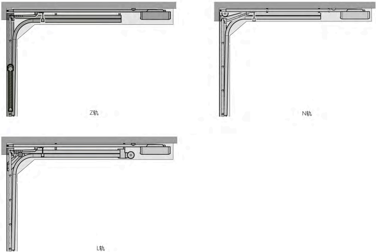
车库门侧面示意图
