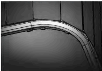
转角地轨榫卯式连接，运行平滑稳定。
